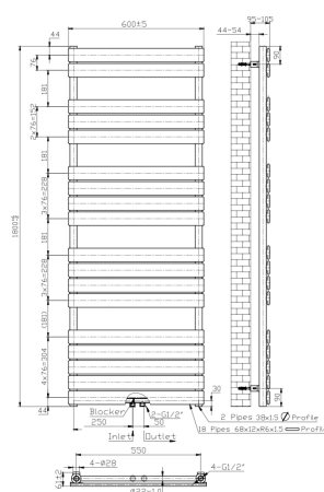
Abgebildet: Ausführung 60 × 180
