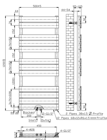
Abgebildet: Ausführung 50 × 120
